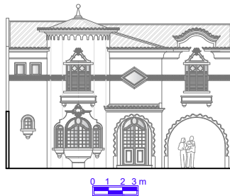
Elevação 01
